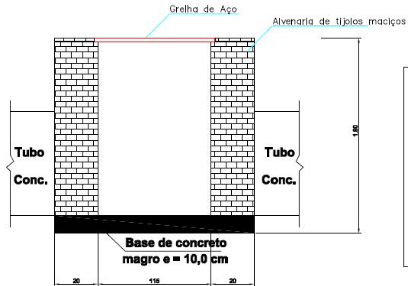
Corte BB' localizada na pista
