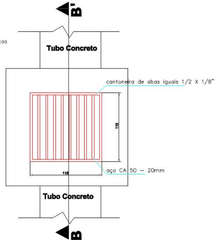
Vista superior (Boca de lobo) localizada na Pista
